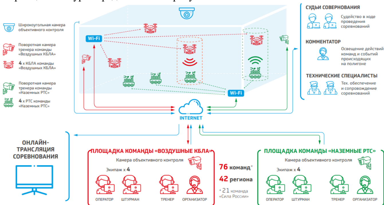
Рисунок 1 – Принципиальная схема полигона для выполнения конкурсного задания этапа «Зарница» Конкурса
